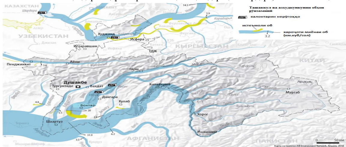
Расми 1. – Иқтидори гидроэнергетикии ҳавзаҳои дарёҳои Сирдарё, Вахш ва Панҷ
