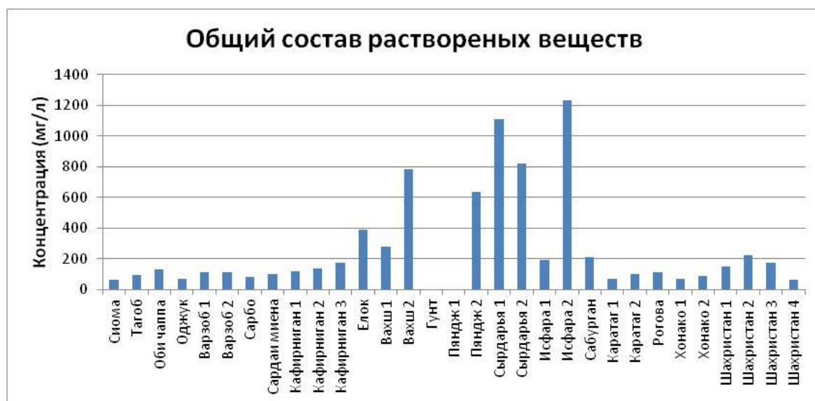
Рисунок 3. Общий состав растворенных в водах веществ в реках
