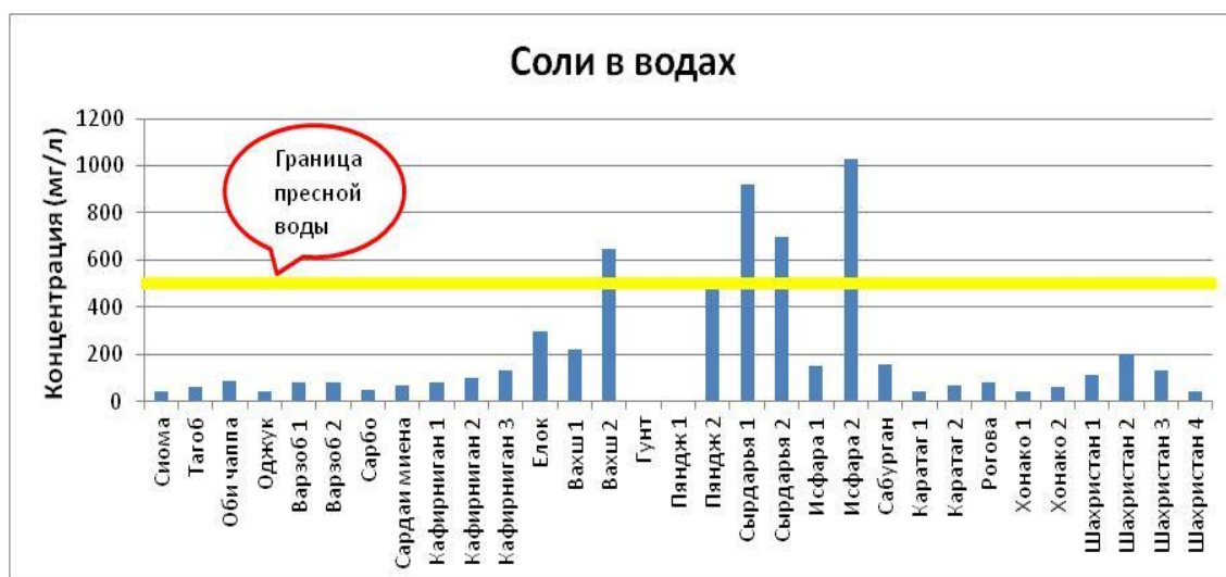
Рисунок 2. Концентрация солей в реках Таджикистана
