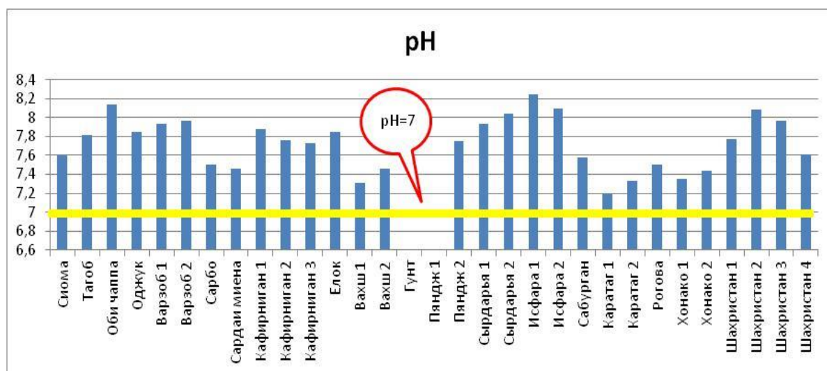
Рисунок 1. рН характеристика вод в реках Таджикистана в период половодья
